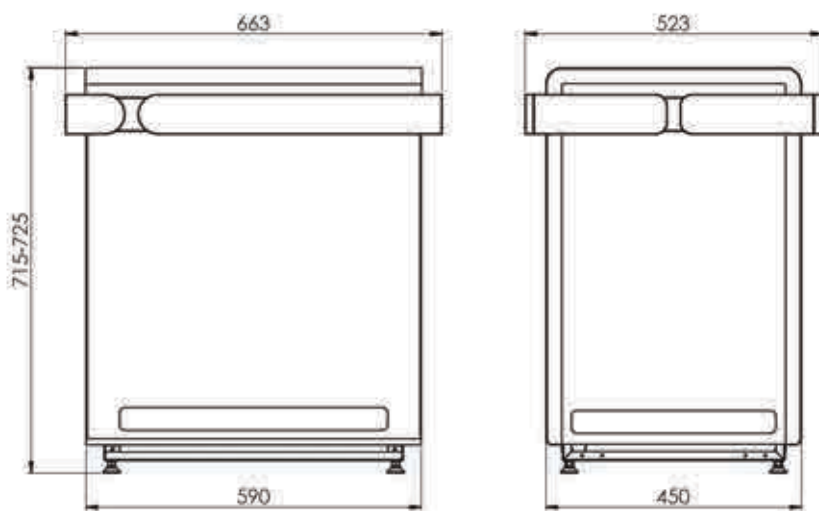
Obr. 6 Rozměry modelu Concept R 12 kW a 15 kW (CP-R-120 / CP-R-150 / CP-RB-120 / CP-RB-150) Rozměry v mm
