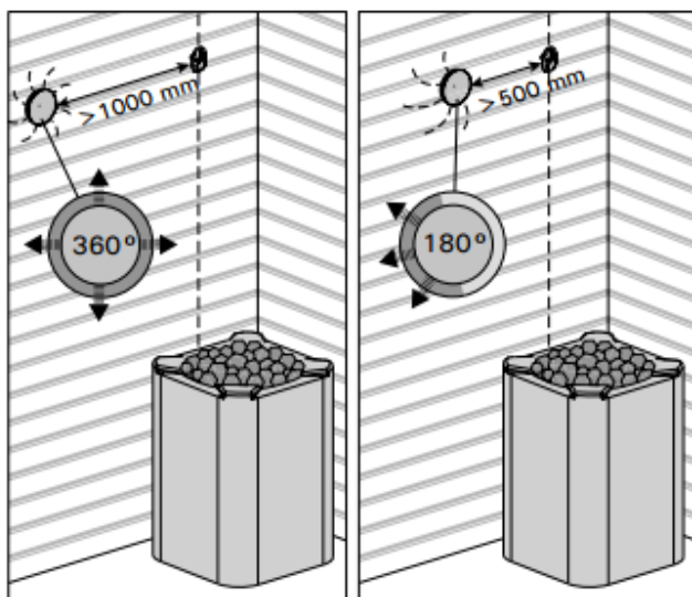
Figure 10. Sensor's minimum distance from an air vent Obrazek 10. Minimalní rozmery pro umístění čidla
