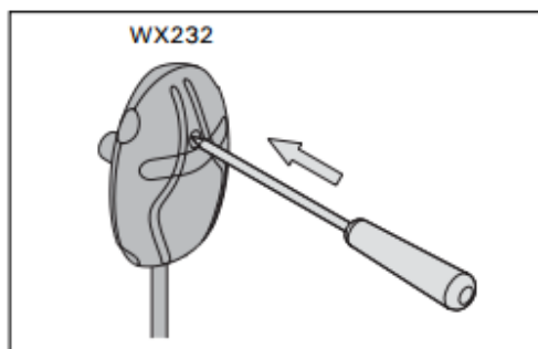
Figure 11. Reset button of the overheat protector Obrazek 11. Reset tlačítko tepelné ochrany
