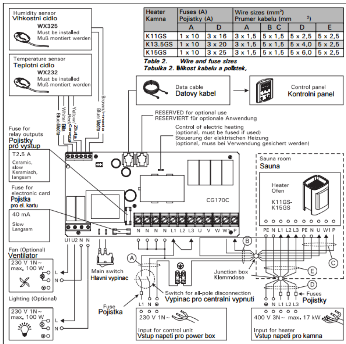
Obrazek 6. Elektrické zapořeni (K11GS–K15GS)
