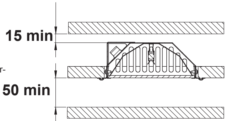
Abb. 2 - Mindestabstände Wandmontage
